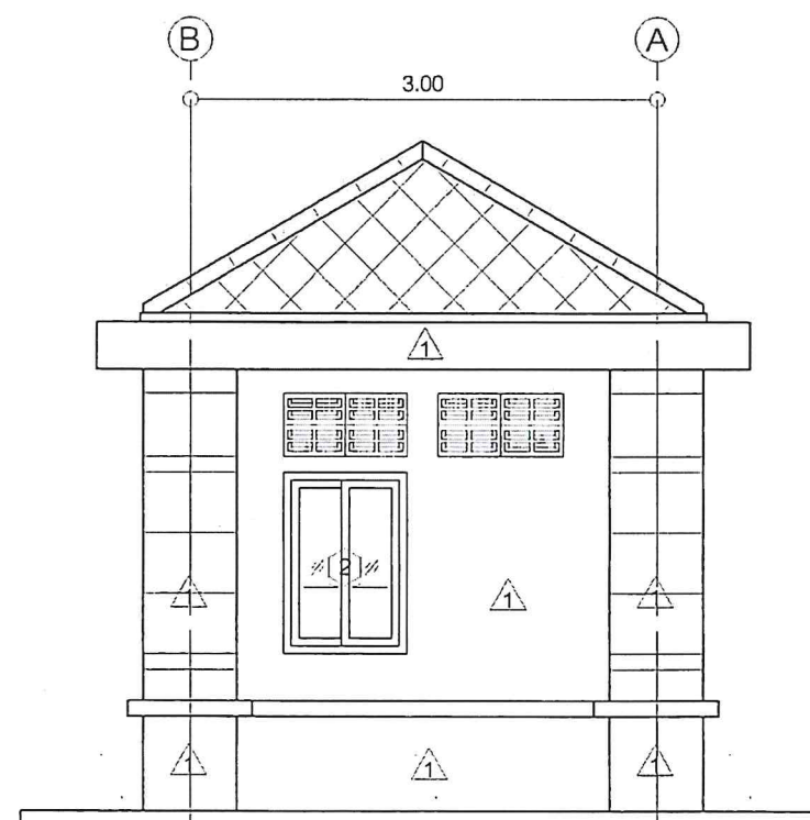
รูปด้าน 4
