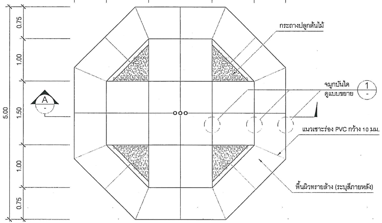
แปลนเสาธง
