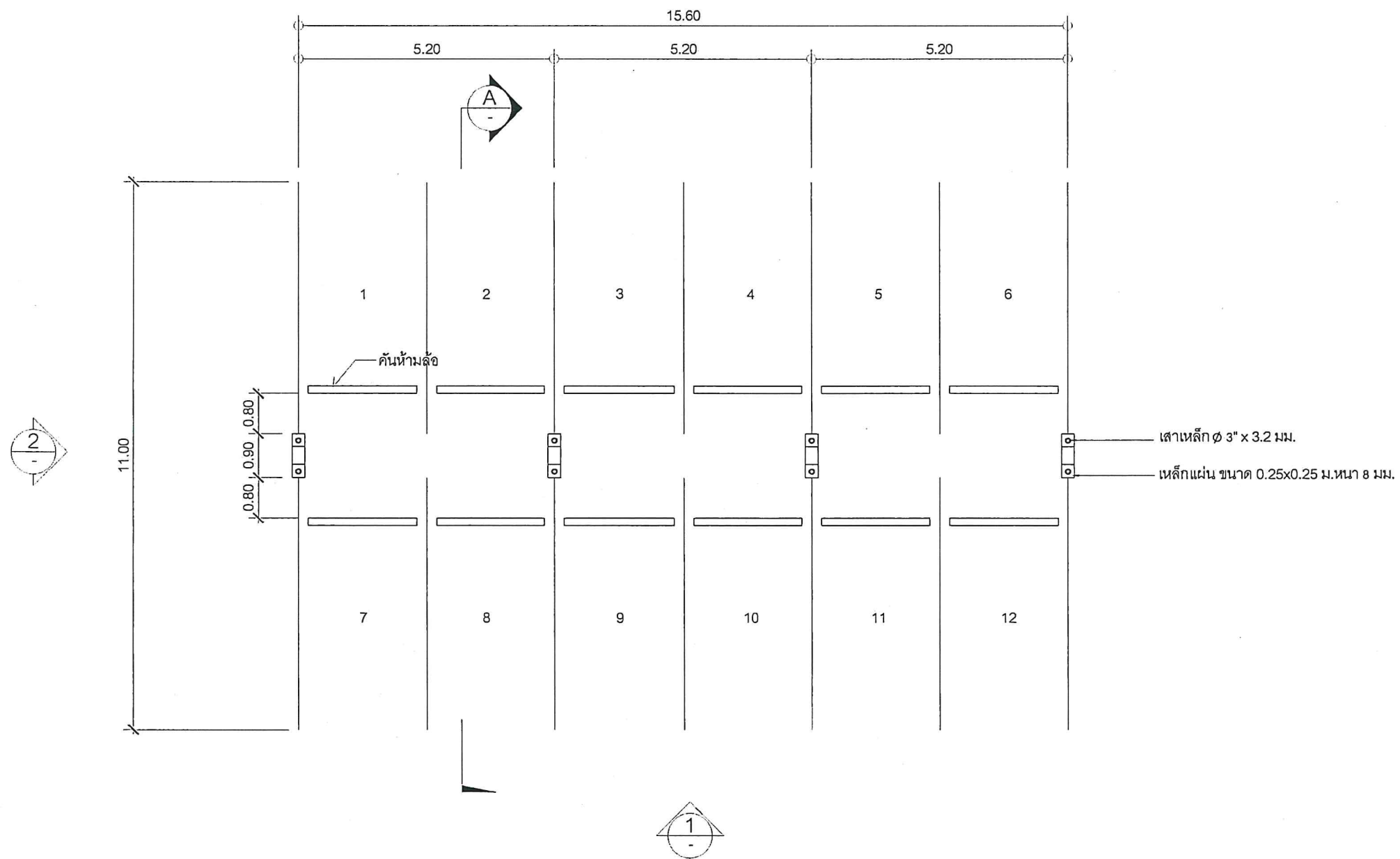
แปลนพื้นโรงจอดรถยนต์ มาตราส่วน 1:100
