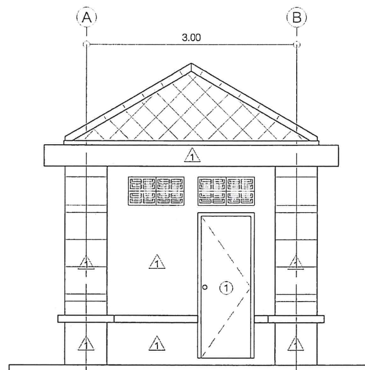
รูปด้าน 2
