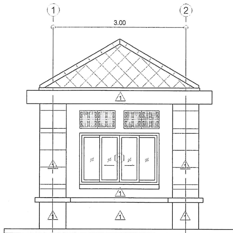
รูปด้าน 1
