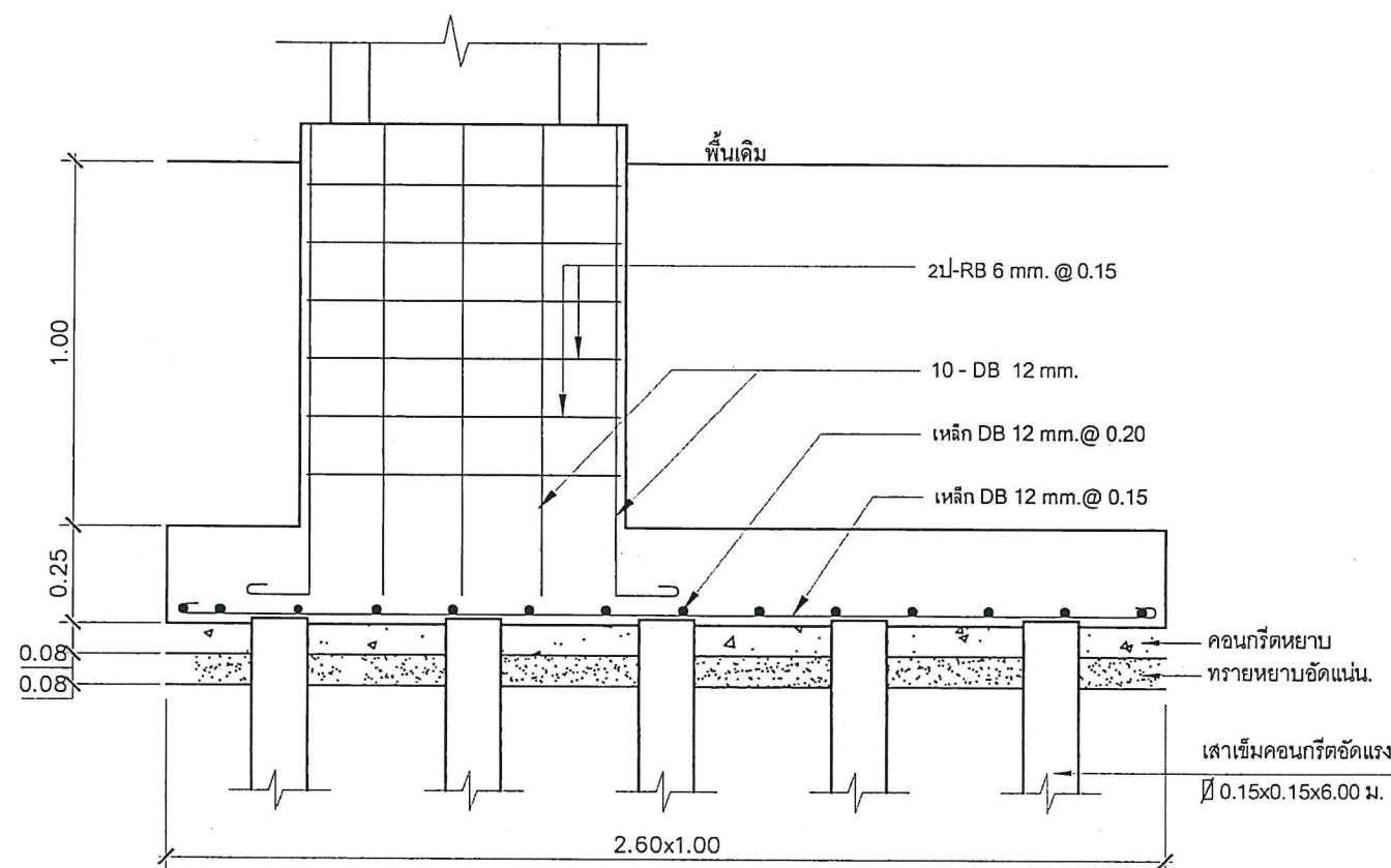
ขยายฐานราก มาตราส่วน 1:20
