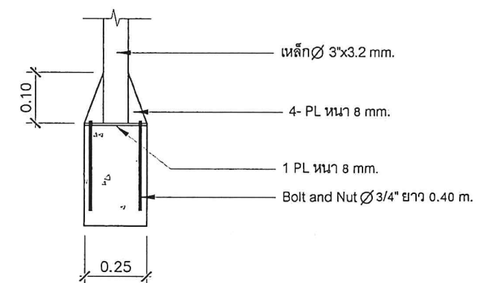
ขยายการเชื่อมเสา มาตราส่วน 1:20
