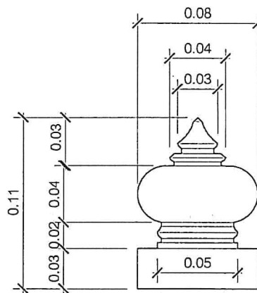
หัวเม็ดทองเหลืองกลิ้ง
