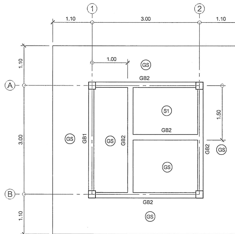
แปลนเสา คาน และพื้น
