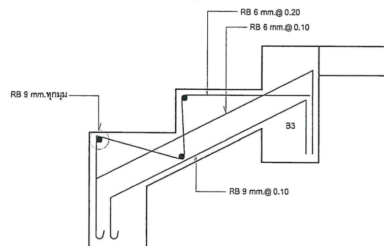
แบบขยายโครงสร้างบันได 1
