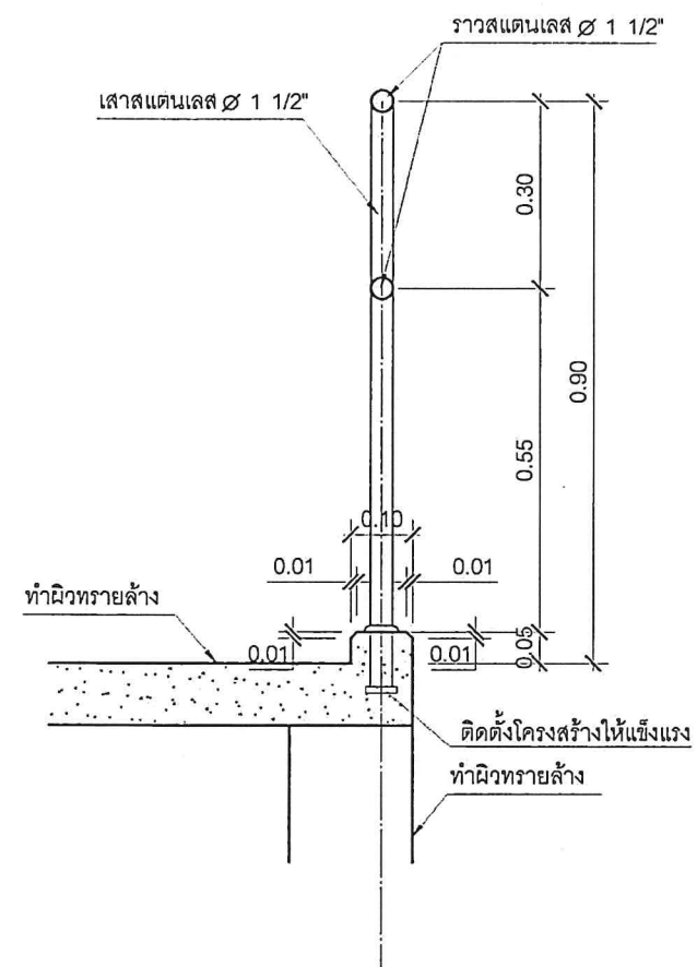
แบบขยายราวกันตก
