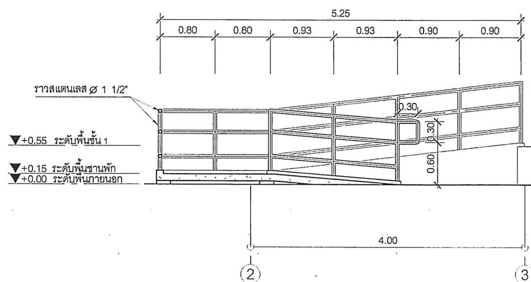
รูปตัด A
