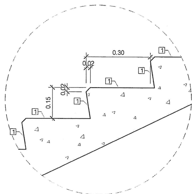
แบบขยายรายละเอียดบันได 1
